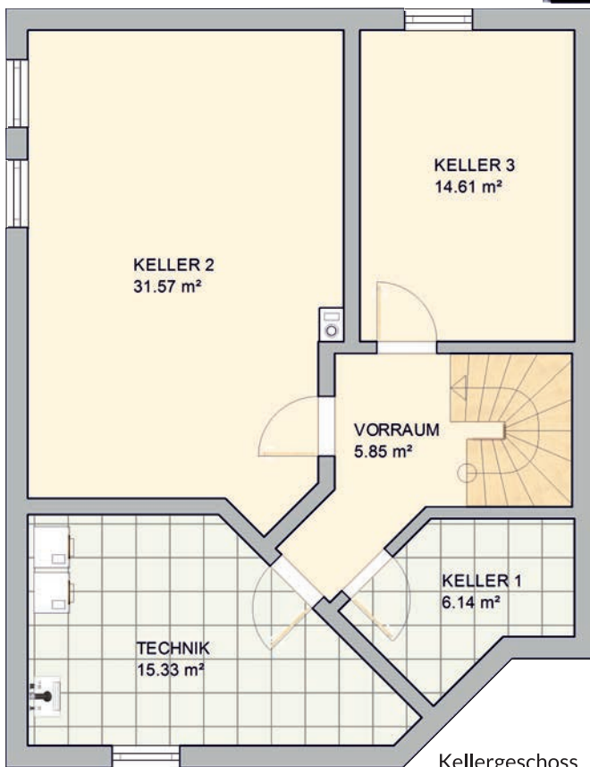
Kellergeschoss
