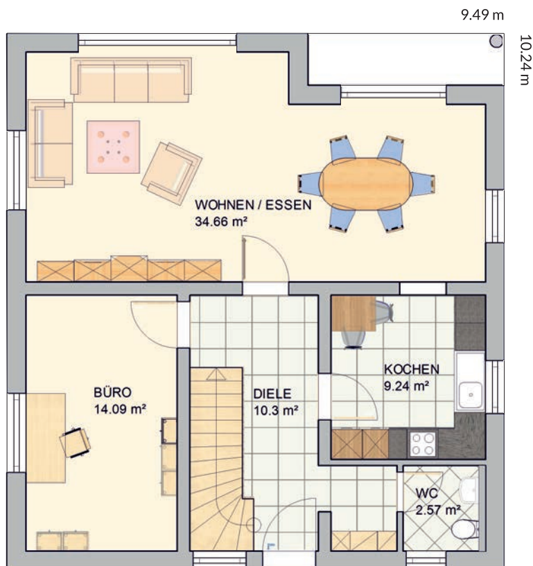
Erdgeschoss
