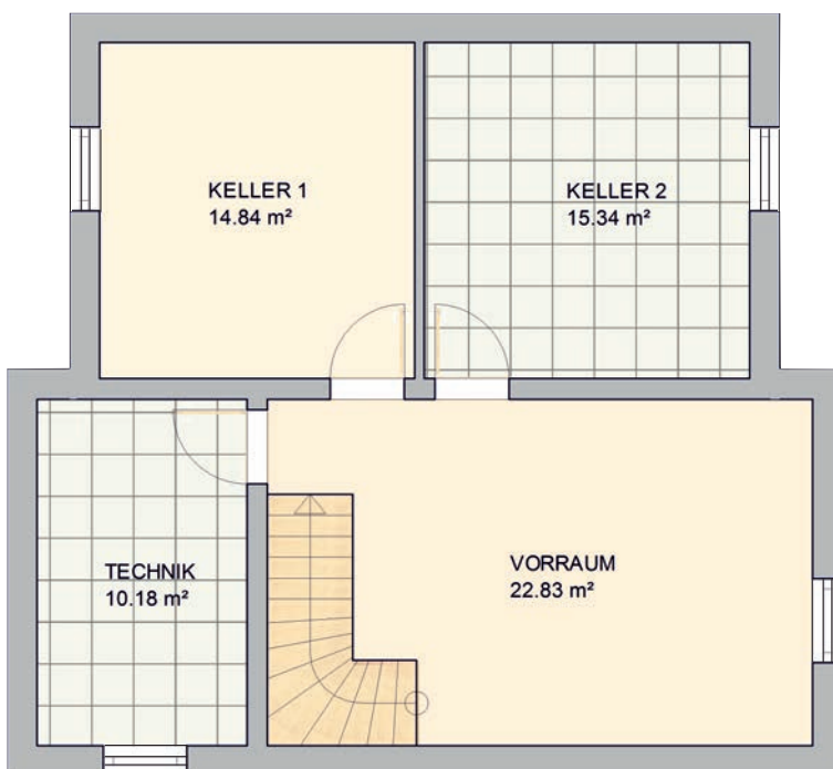
Kellergeschoss
